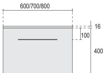
Predný pohľad
